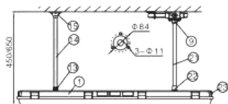
Pendant type-Up wiring
