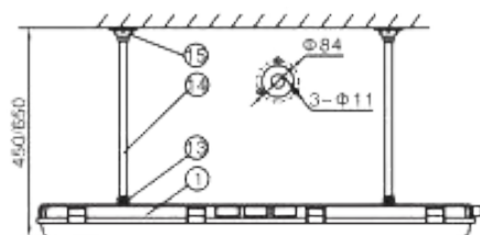
Pendant type-Side wiring
