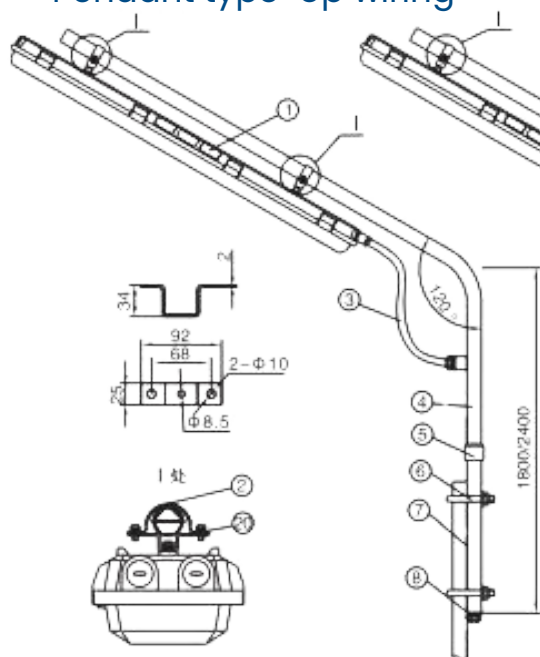
Pendant type-Up wiring
